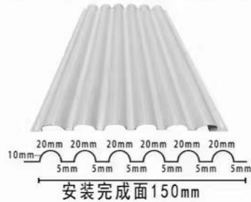
150面20+5半圆长城板
