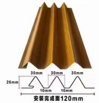
120面W型长城板
